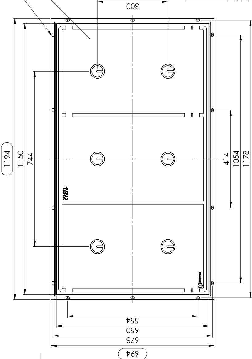
Draufsicht / Top view Variante B / Version B
