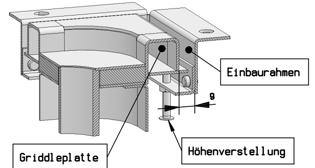
Detail Griddleplatte + Einbaurahmen
