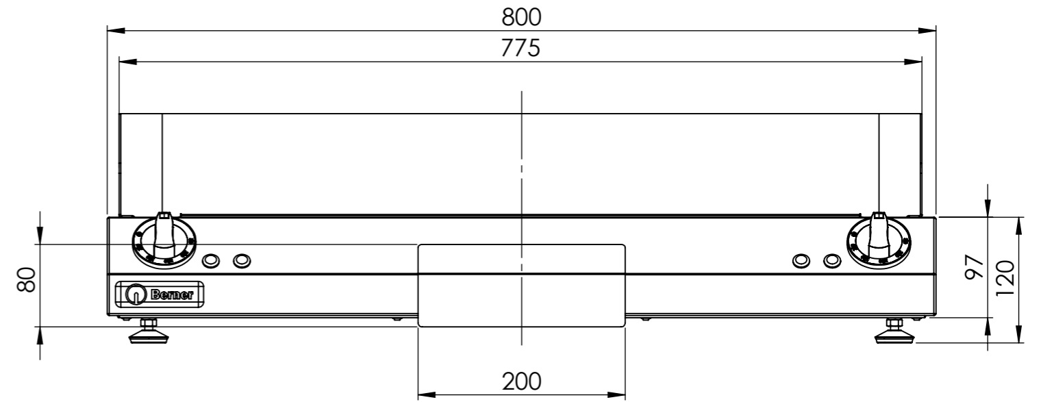
Vorderansicht / Front view
