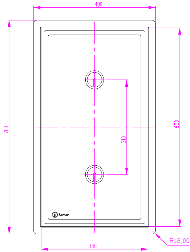
Generatoransicht generator view
