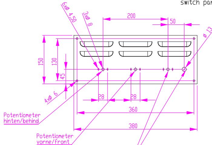
Hauptschalter mit Betriebsleuchte grün 230V main switch with green lamp for starting 230V
