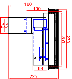
Generatoransicht Version Generator Modul Seitenansicht
