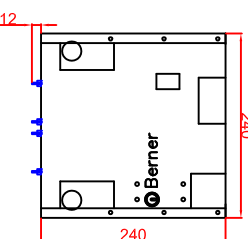
Generatoransichten Version Generator-Spule getrennt Seitenansicht
