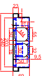
Draufsicht
