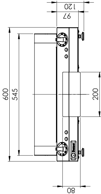
Vorderansicht / Front view
