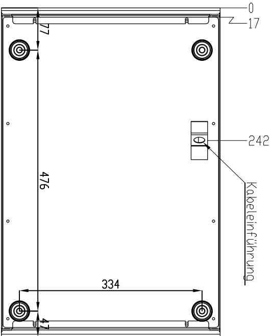
Unteransicht
