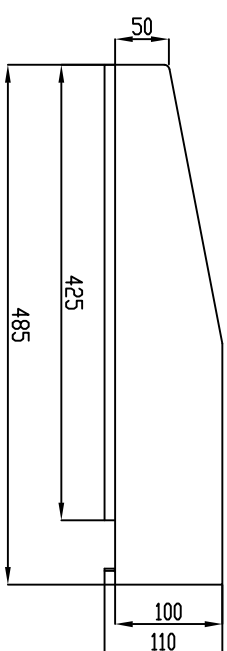
optional: Spritzschutz
