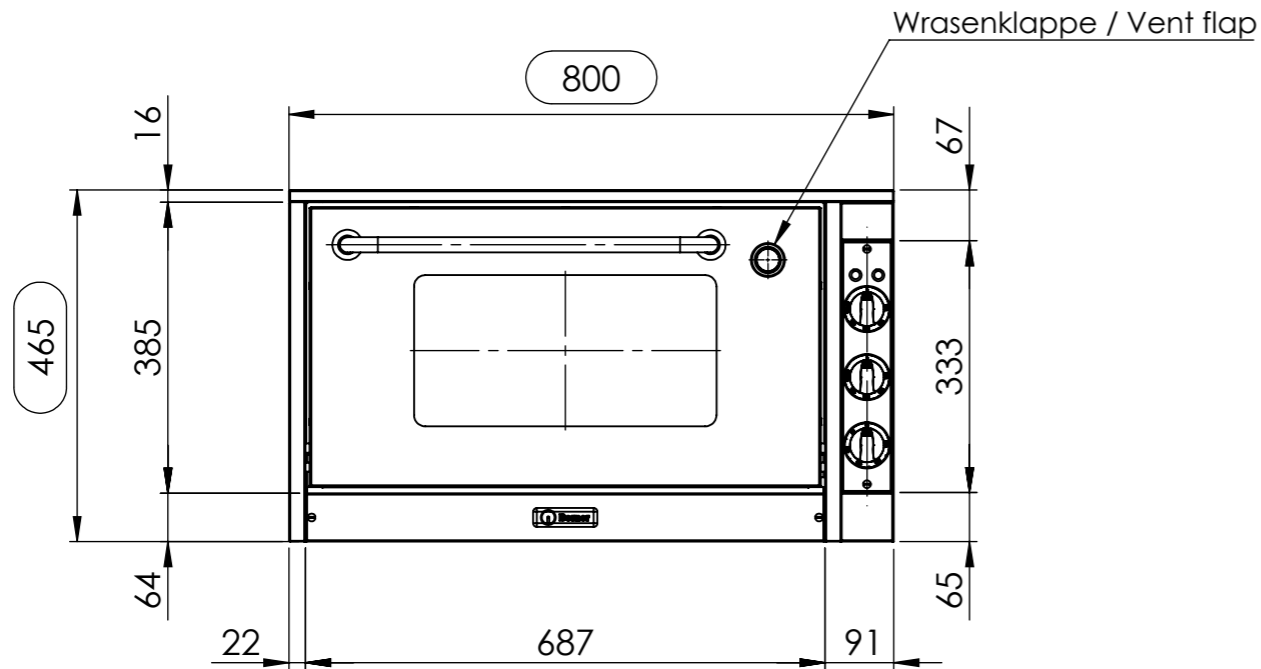
Vorderansicht / Front view
