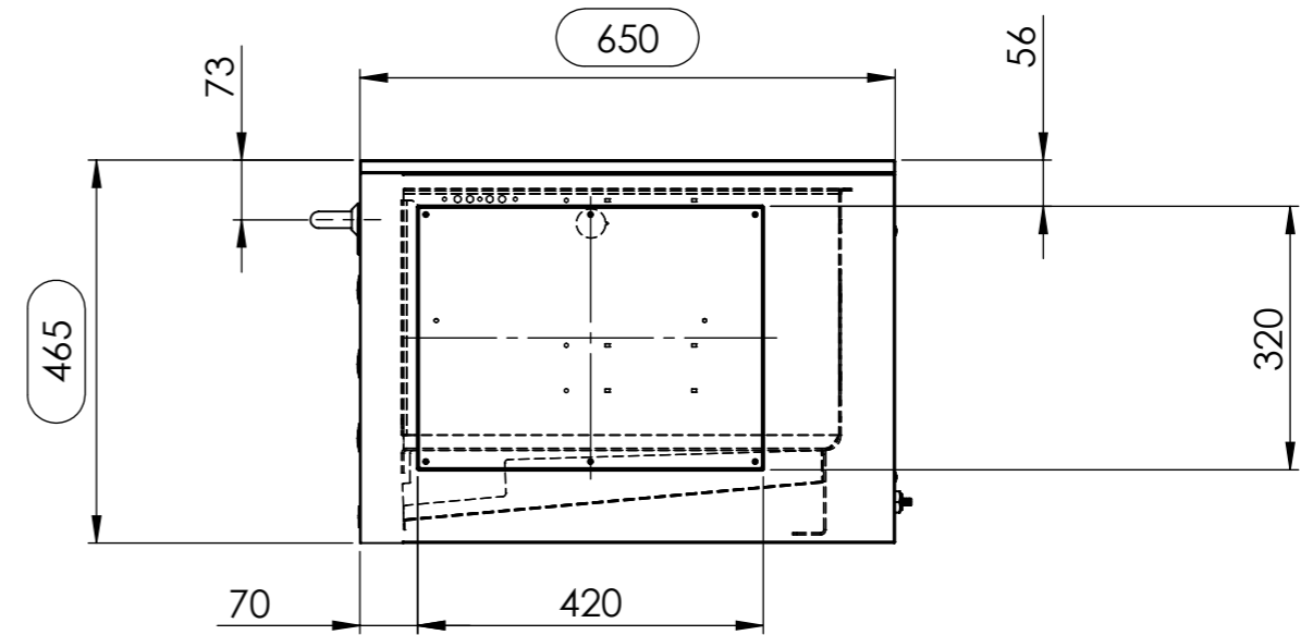
Seitenansicht / Side view
