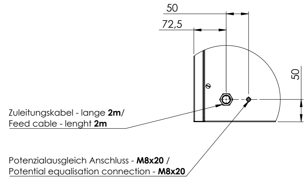
Detailansicht - Rückseite / Detail view - back side
