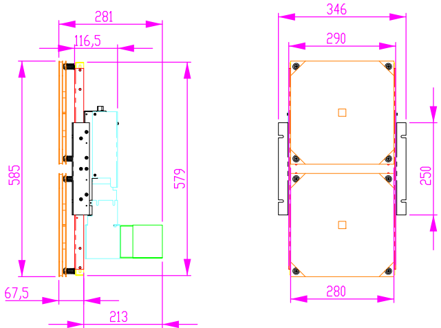
Generatoransicht generator view
