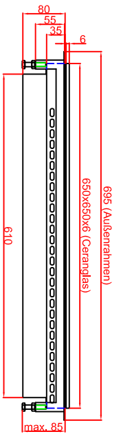
Variante "B" Ausschnitt in Abdeckung flächenbündiger Einbau 658mm x 658mm
