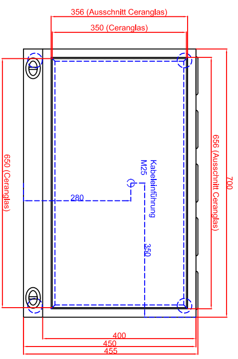
Draufsicht
