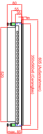
Variante "B" Ausschnitt in Abdeckung flächenbündiger Einbau 358mm x 568mm
