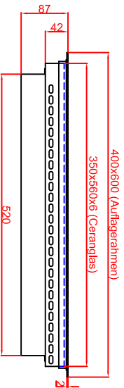
Variante "A" Ausschnitt in Abdeckung Einbau mit Auflagerahmen 380mm x 585mm
