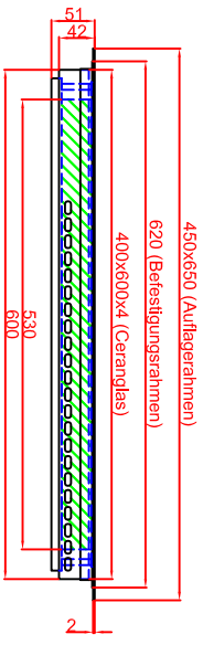
Variante "A" Ausschnitt in Abdeckung Einbau mit Auflagerahmen 430mm x 630mm
