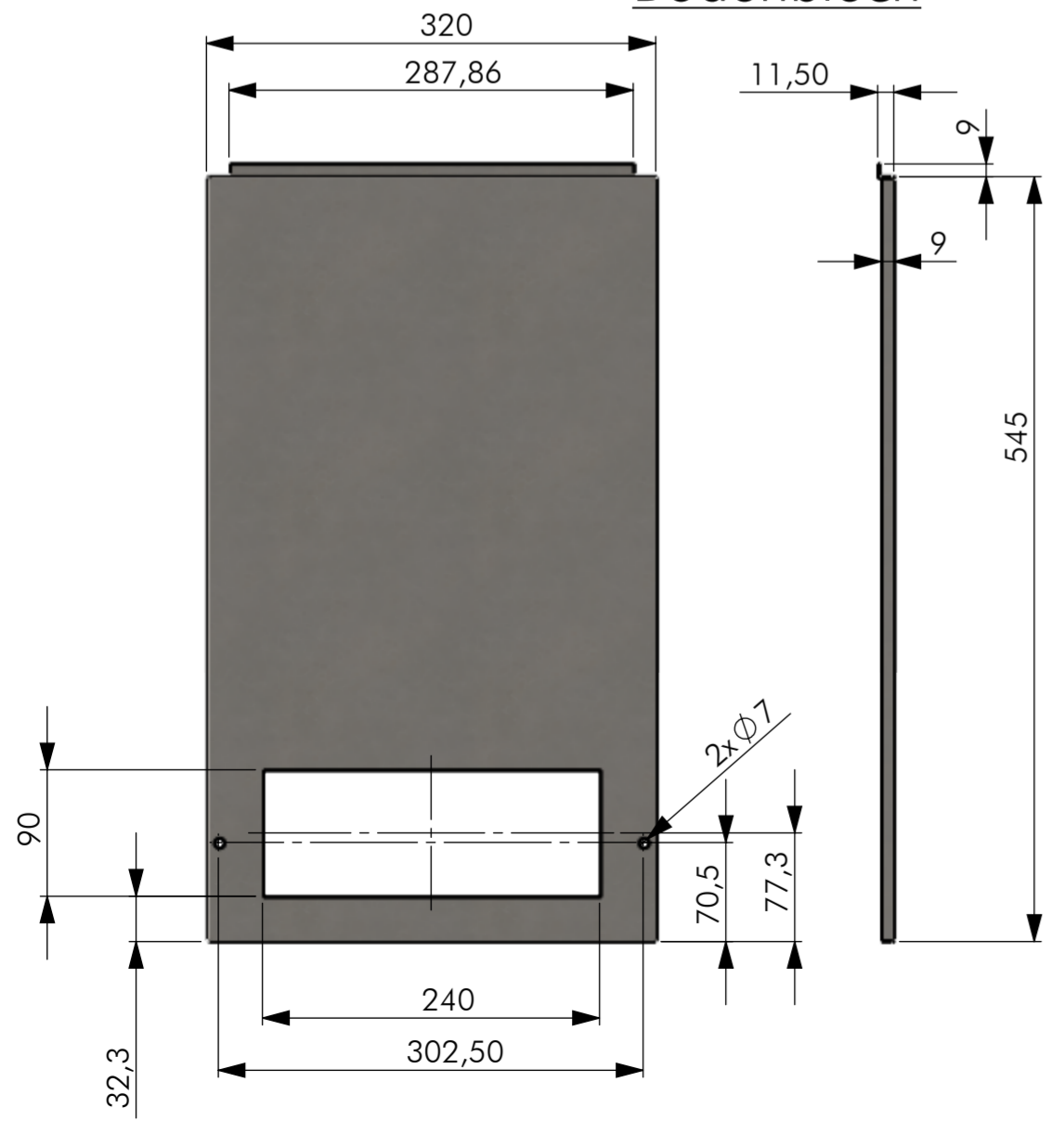
Bodenblech
