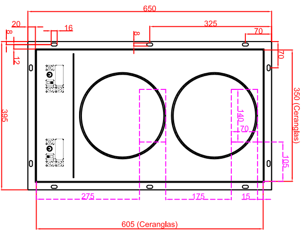
Ausschnitt in Abdeckung 356mm x 611mm Ansicht mit Luftschachtöffnungen
