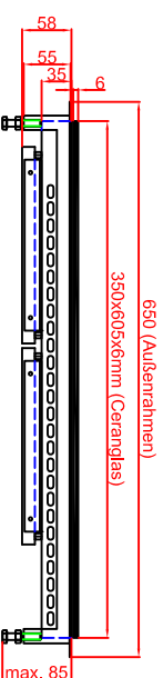
Ausschnitt in Abdeckung 356mm x 611mm Version Generator-Spule getrennt
