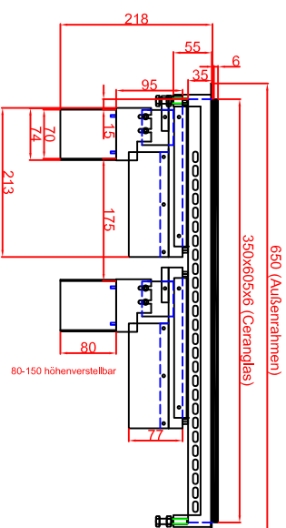
Ausschnitt in Abdeckung 356mm x 611mm Version Generator Modul angebaut
