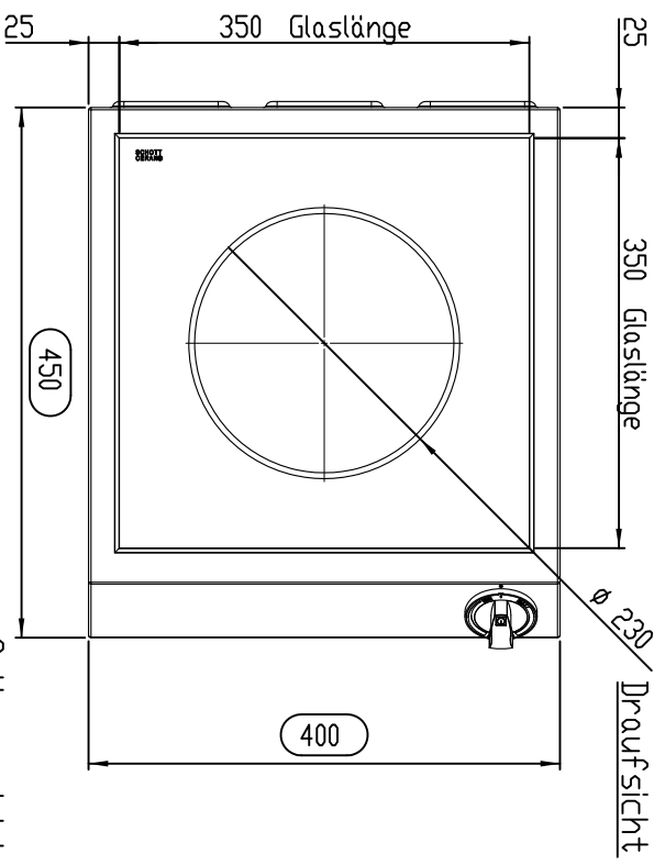
Draufsicht
