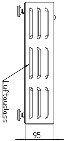
Rückansicht
