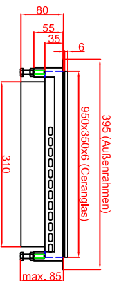
Variante "B" Ausschnitt in Abdeckung flächenbündiger Einbau 958mm x 358mm
