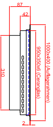
Variante "A" Ausschnitt in Abdeckung Einbau mit Auflagerahmen 980mm x 380mm
