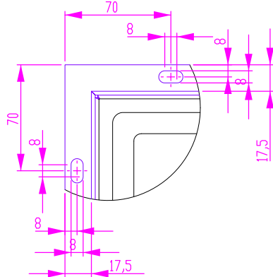
DETAIL A MAßSTAB 2 : 5
