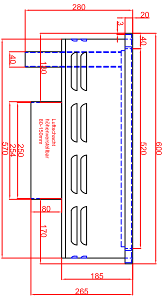
Seitenansicht
