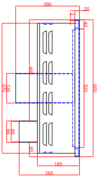
Frontansicht
