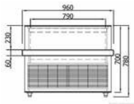
309904 Seitenskizze
