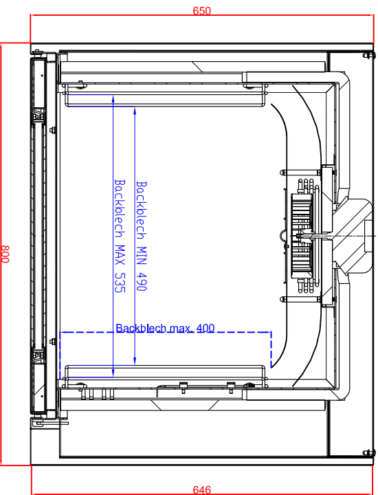
Draufsicht
